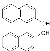
BINOL
